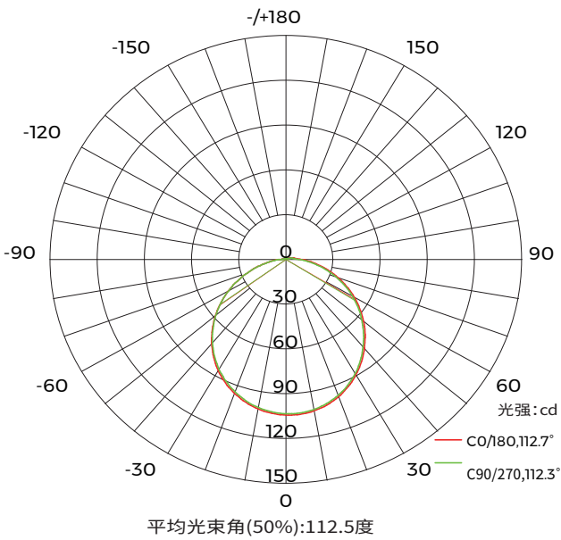
配光曲线
